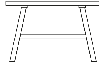
CONSOLE TABLE H: 780 W: 1200 D: 400
