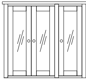
4' 6" GLASS DOOR DRESSER TOP H 1230 W: 1377 D: 315
